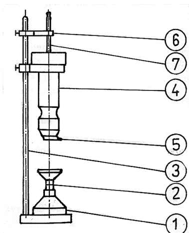
Obr.:Schéma viskozimetra
