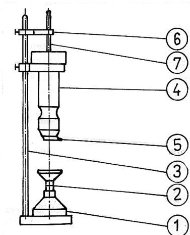
Obr.:Schéma viskozimetra
