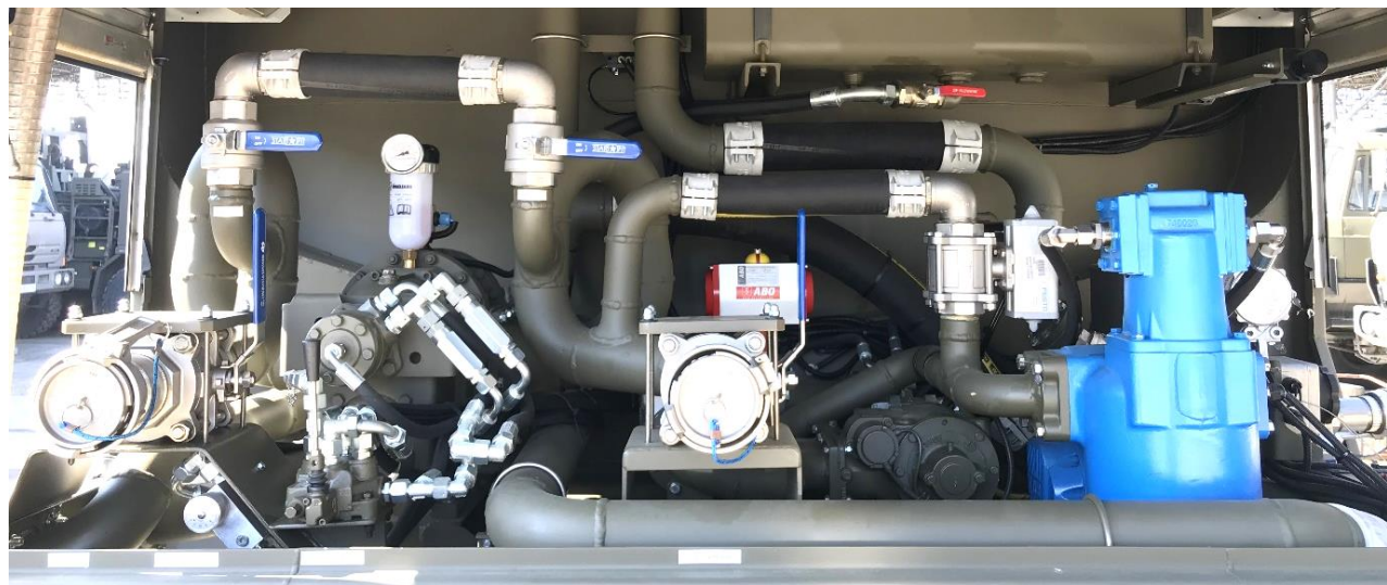
Obrázok 28. Spojenia v technologickej skrini [11]
