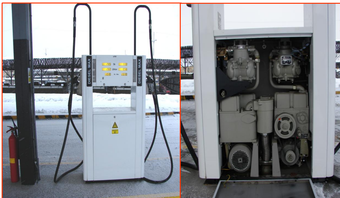
Obrázok č. 2. a 3. Výdajný stojan typ ADAST ADAMIN 8931.50/E/SK
